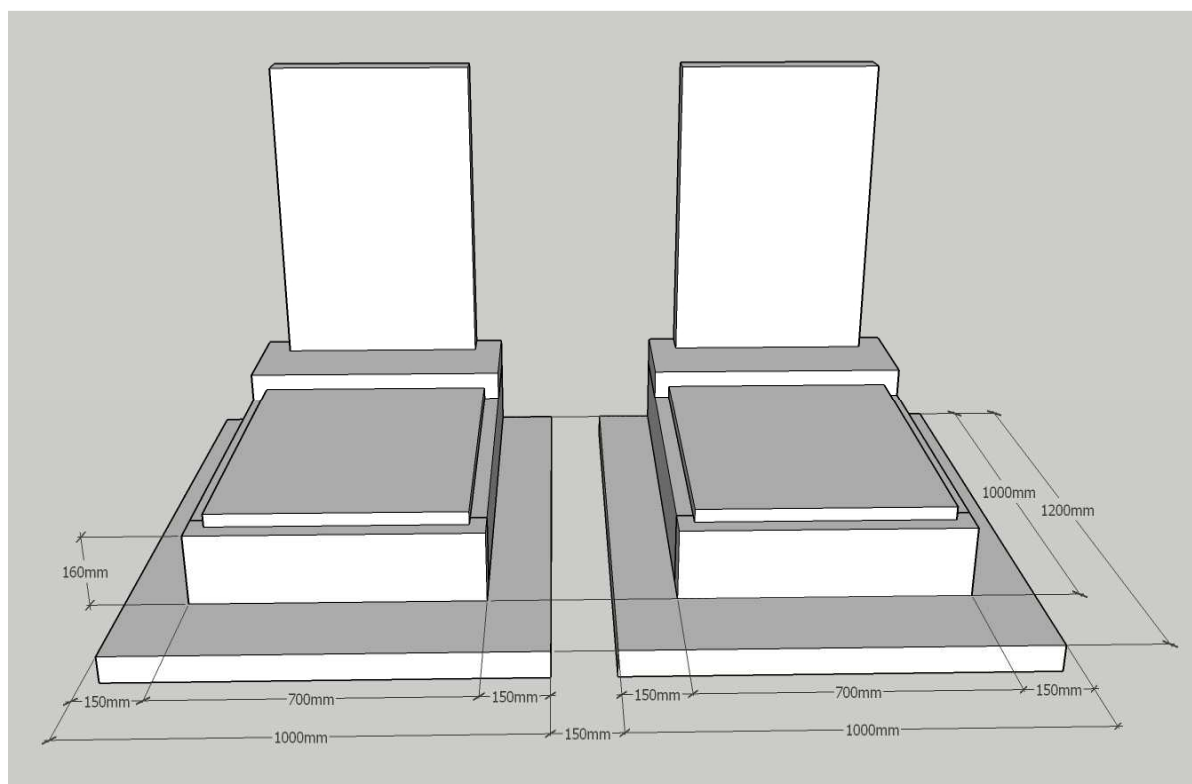
Obr. 1 (rozměry rámu a ochozu)
